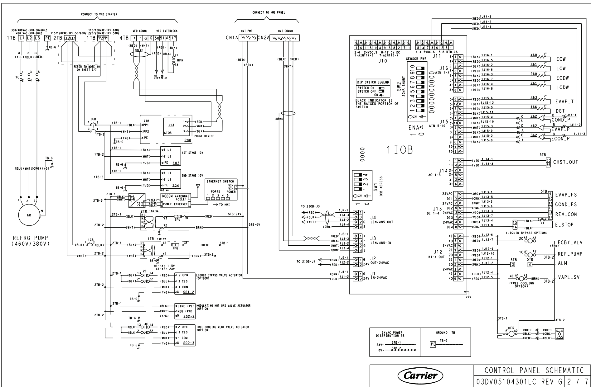
Fig. 23 — IOB1
